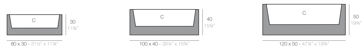
JARDINERA 80 x 30 cm JARDINIERE 31 1/2" x 11 3/4"
