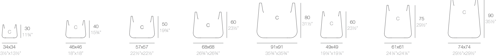
34x34 13½"x13½" 46x46 18"x18" 57x57 22½"x22½" 68x68 26¾"x26¾" 91x91 35¾"x35¾" 49x49 19¾"x19¾" 61x61 24¼"x24¼" 74x74 29½"x29½" ULM cuadrada 34 cm ULM square 13½" ULM cuadrada 46 cm ULM square 18" ULM cuadrada 57 cm ULM square 22½" ULM cuadrada 68 cm ULM square 26¾" ULM cuadrada 91 cm ULM square 35¾" ULM cuadrada alta 49 cm ULM square high 19¾" ULM cuadrada alta 61 cm ULM square high 24¼" ULM cuadrada alta 74 cm ULM square high 29½"
