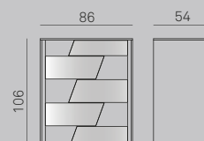
Elemento 5 cassetti P=547 H=1069
