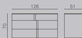
Elemento 3 cassetti P=512 H=701
