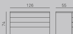
Elemento 4 cassetti P=552 H=742
