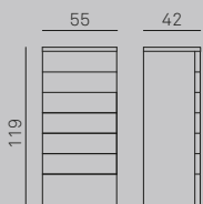
Elemento 7 cassetti P=424 H=1198
