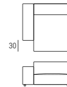
9GY202 Laterale con bracciolo basso Side element with low armrest L130 P130 H66
